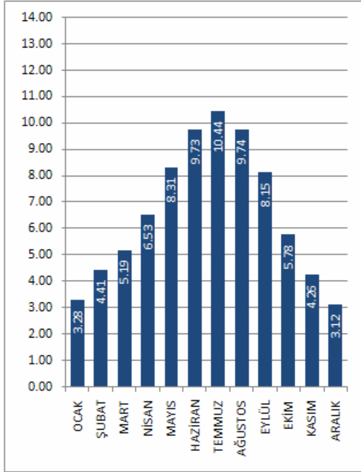
BOLU İLİ GÜNEŞLENME SÜRESİ DEĞERLERİ (Saat)
