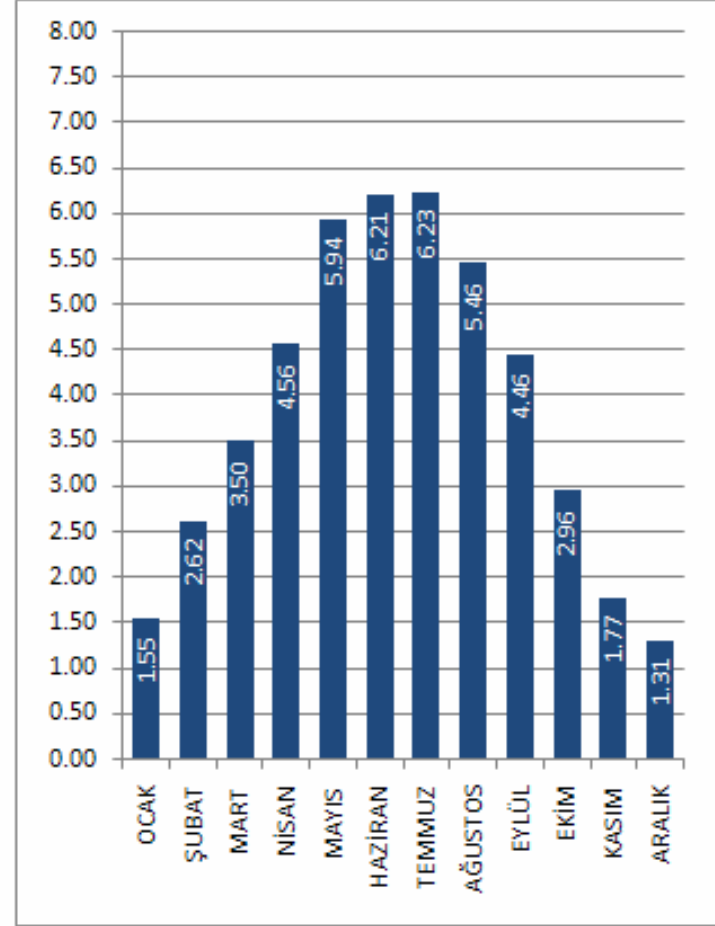
BOLU İLİ GLOBAL RADYASYON DEĞERLERİ (KWh/m 2 -gün)
