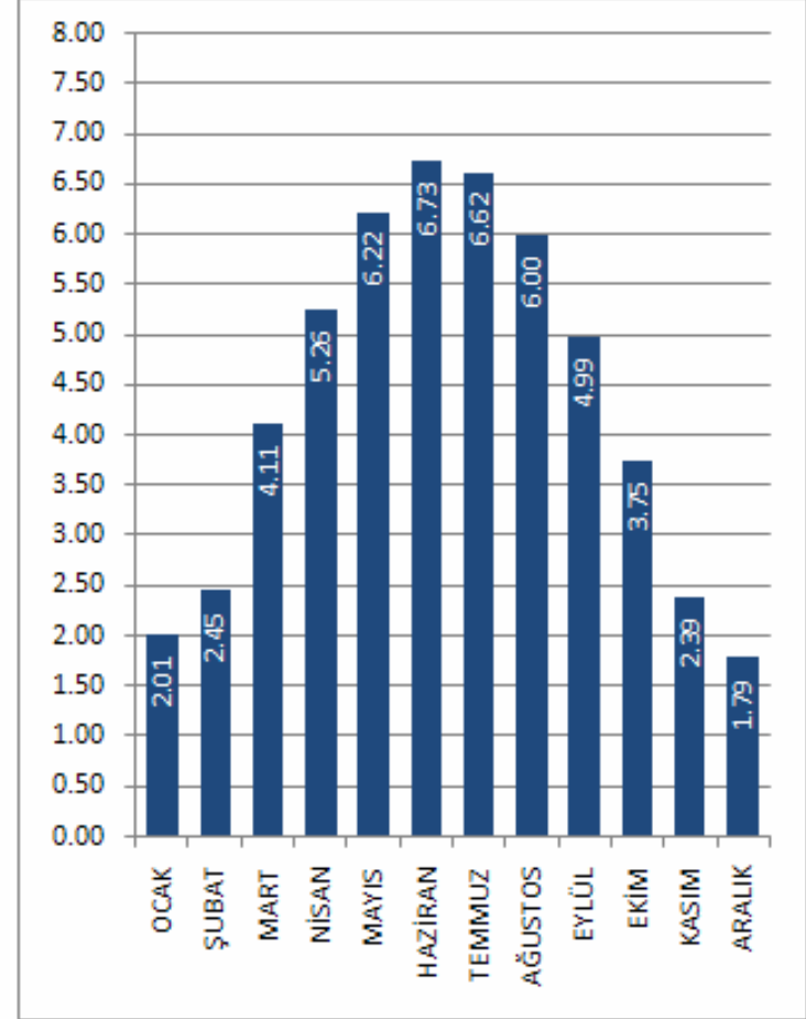
DENİZLİ İLİ GLOBAL RADYASYON DEĞERLERİ (KWh/m 2 -gün)
