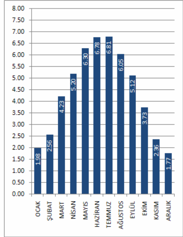
KONYA İLİ GLOBAL RADYASYON DEĞERLERİ (KWh/m 2 -gün)
